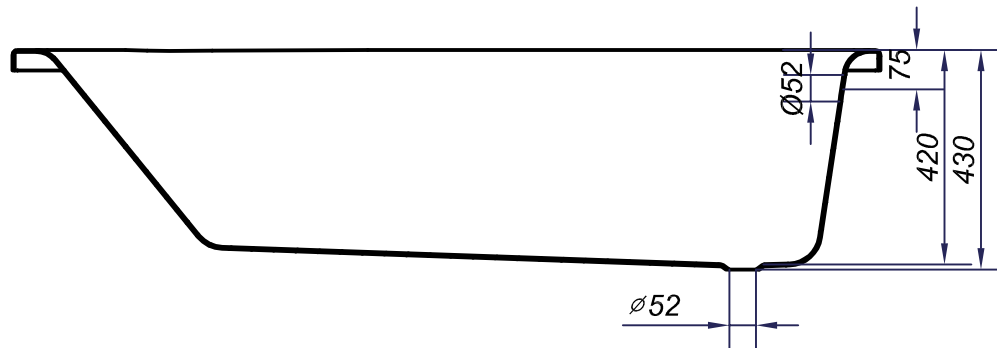
A-A (0,1 : 1)
